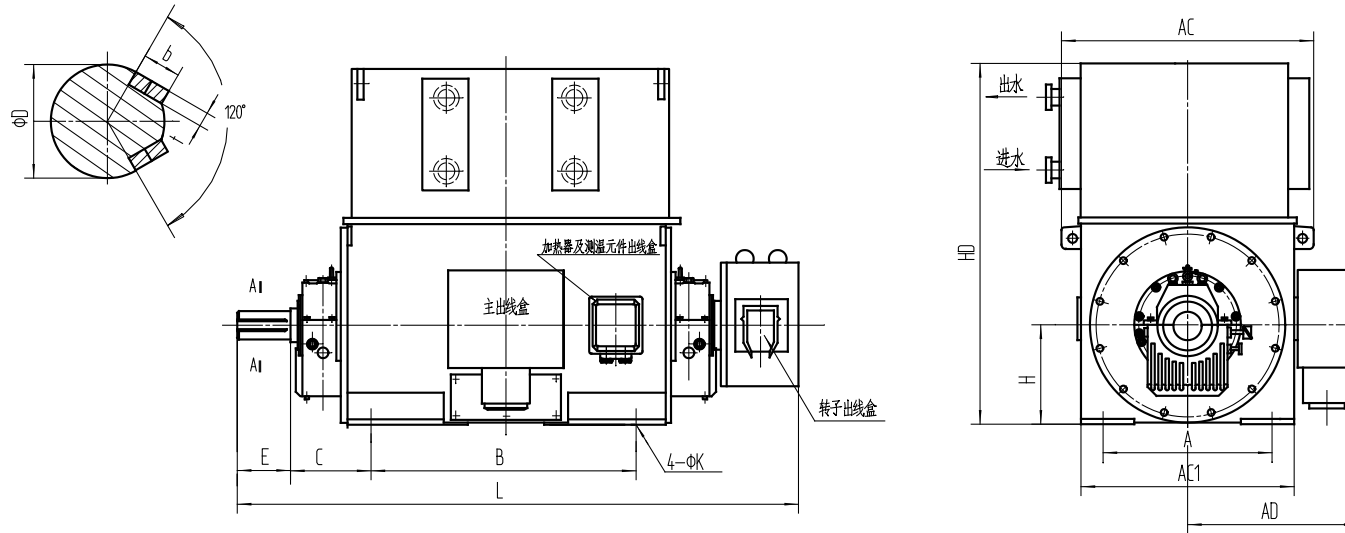
YRKS560-1000 安装尺寸表(6000V) YRKS560-1000 MOUNTING DIMENSIONS TABLE(6000V)
